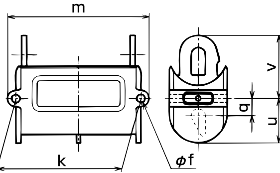
コネクタ
